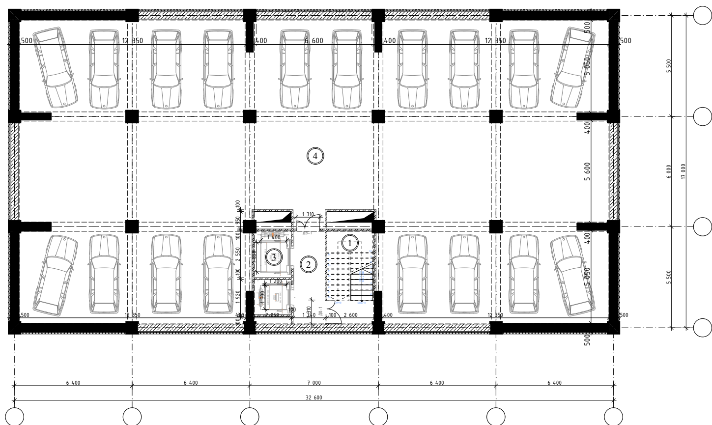
План автопаркинга (Тип-Г)
