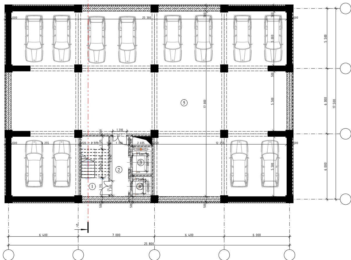
План автопаркинга (Тип-Б)
