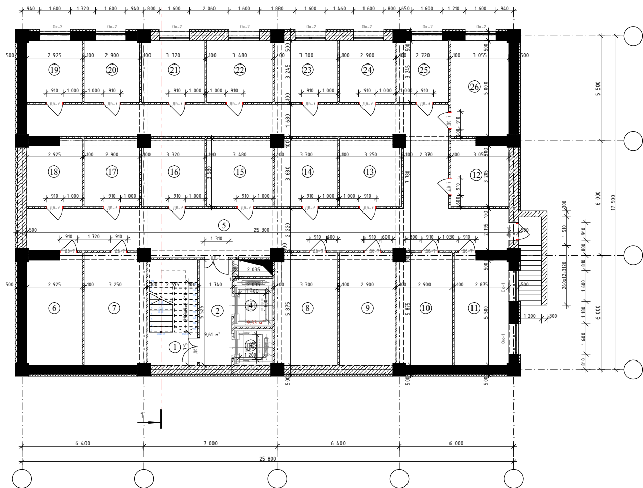
План кладового этажа (Тип-Б)
