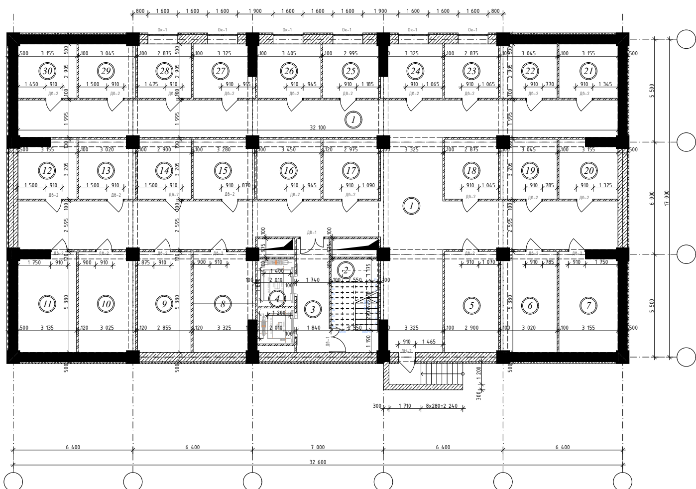
План кладового этажа (Тип-Г)
