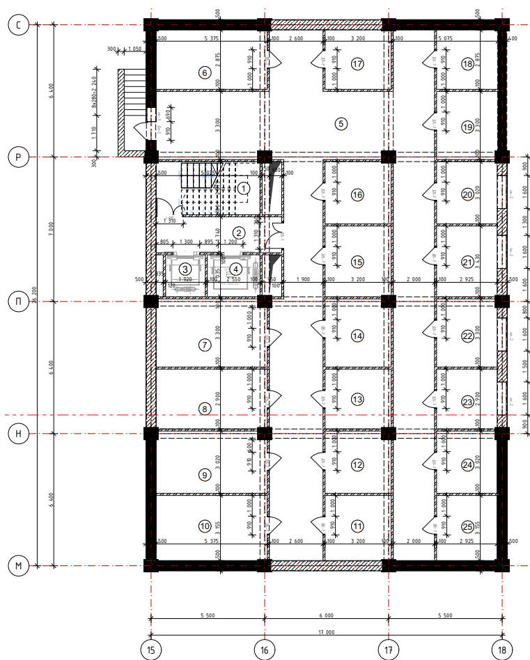
План кладового этажа (Тип-В)
