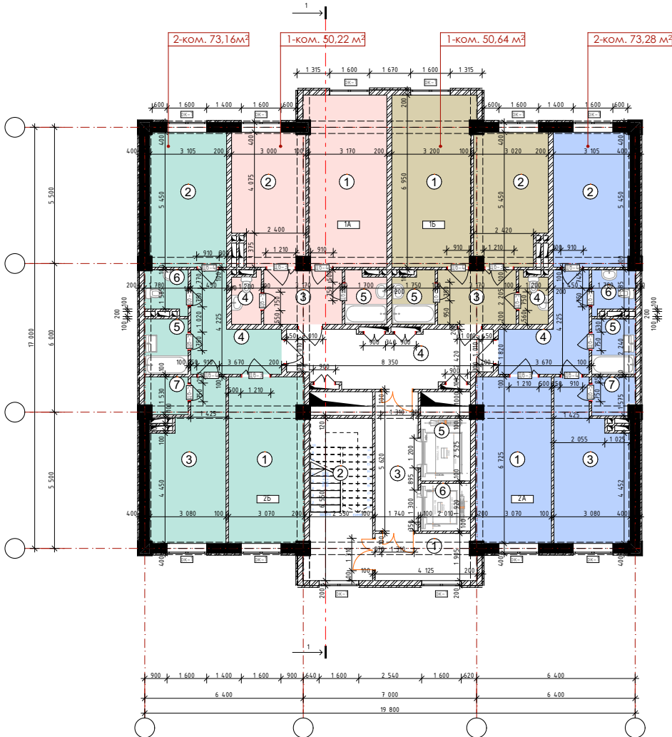
План с 2-го по 12-ый этаж (Тип-А)
