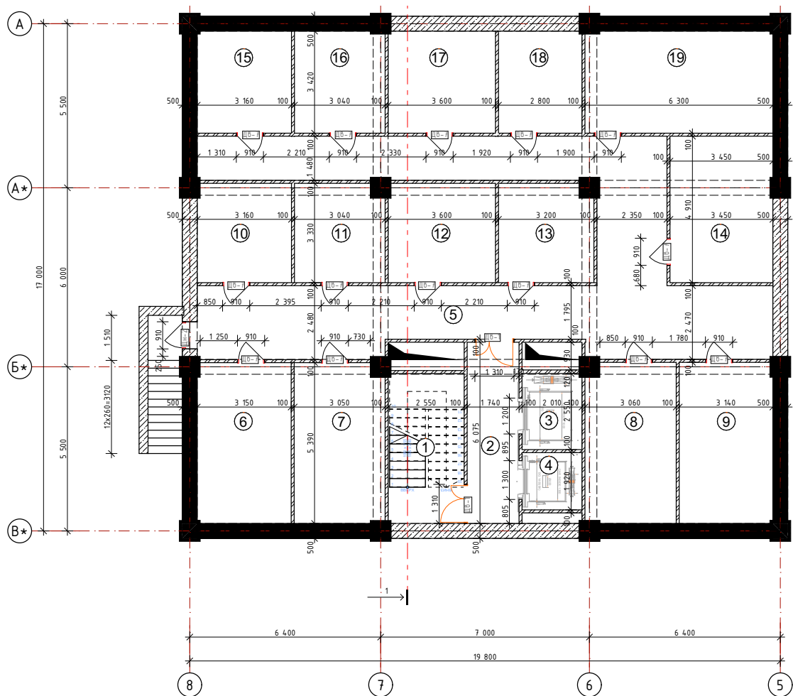
План кладового этажа (Тип-А)
