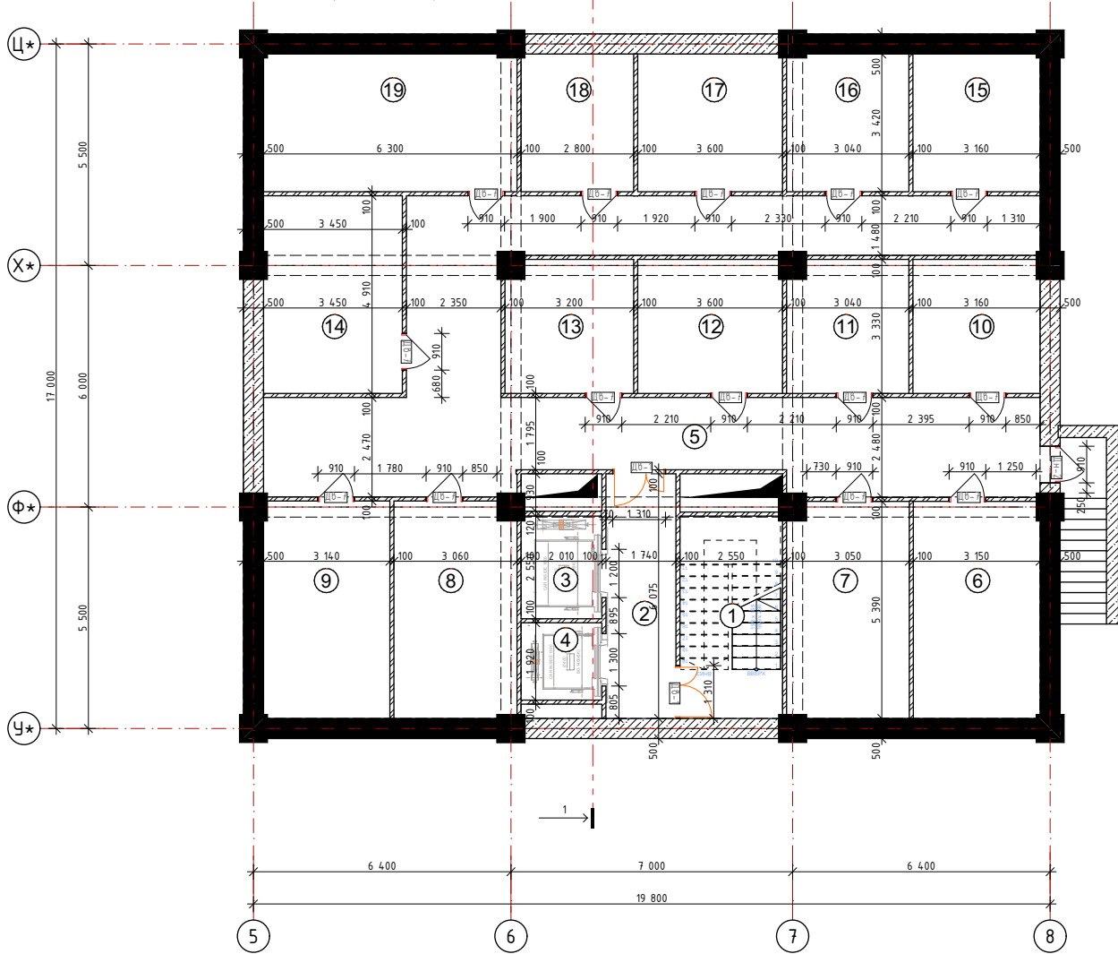
План кладового этажа (Тип-А)
