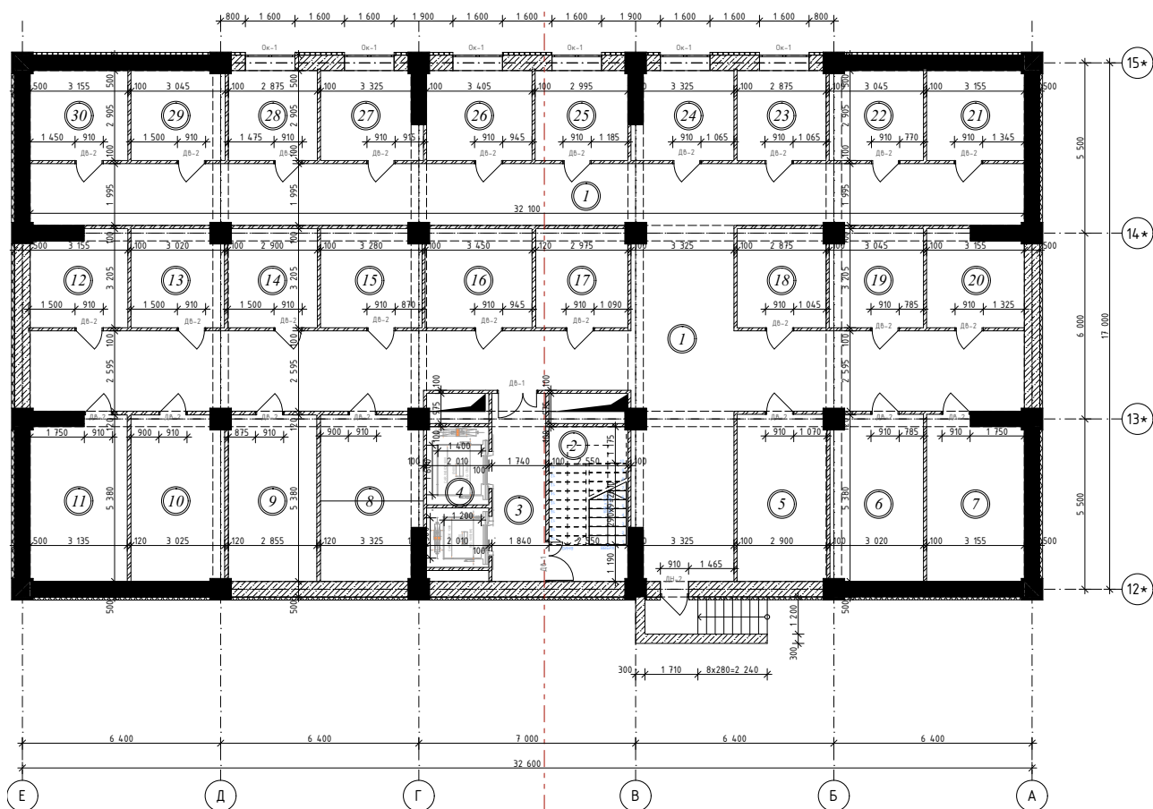
План кладового этажа (Тип-Г)
