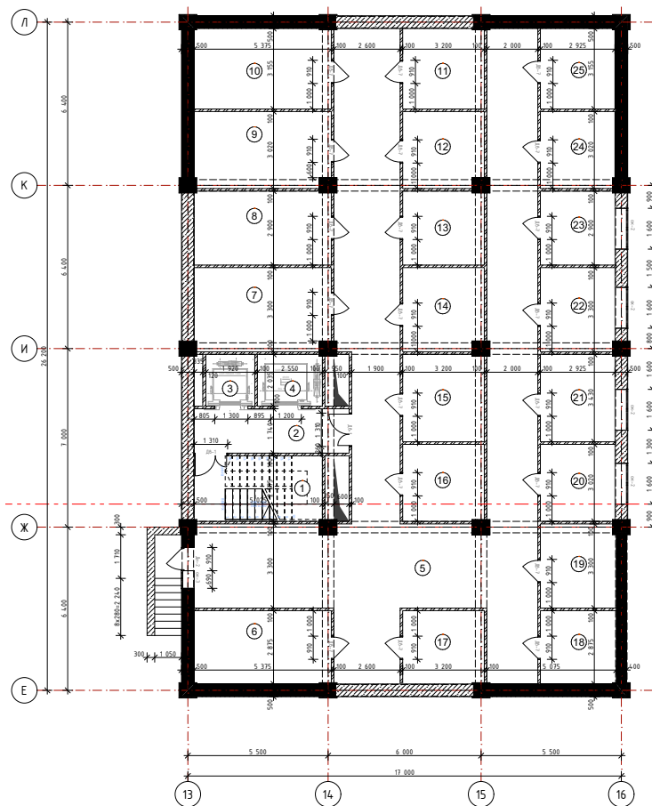
План кладового этажа (Тип-В)
