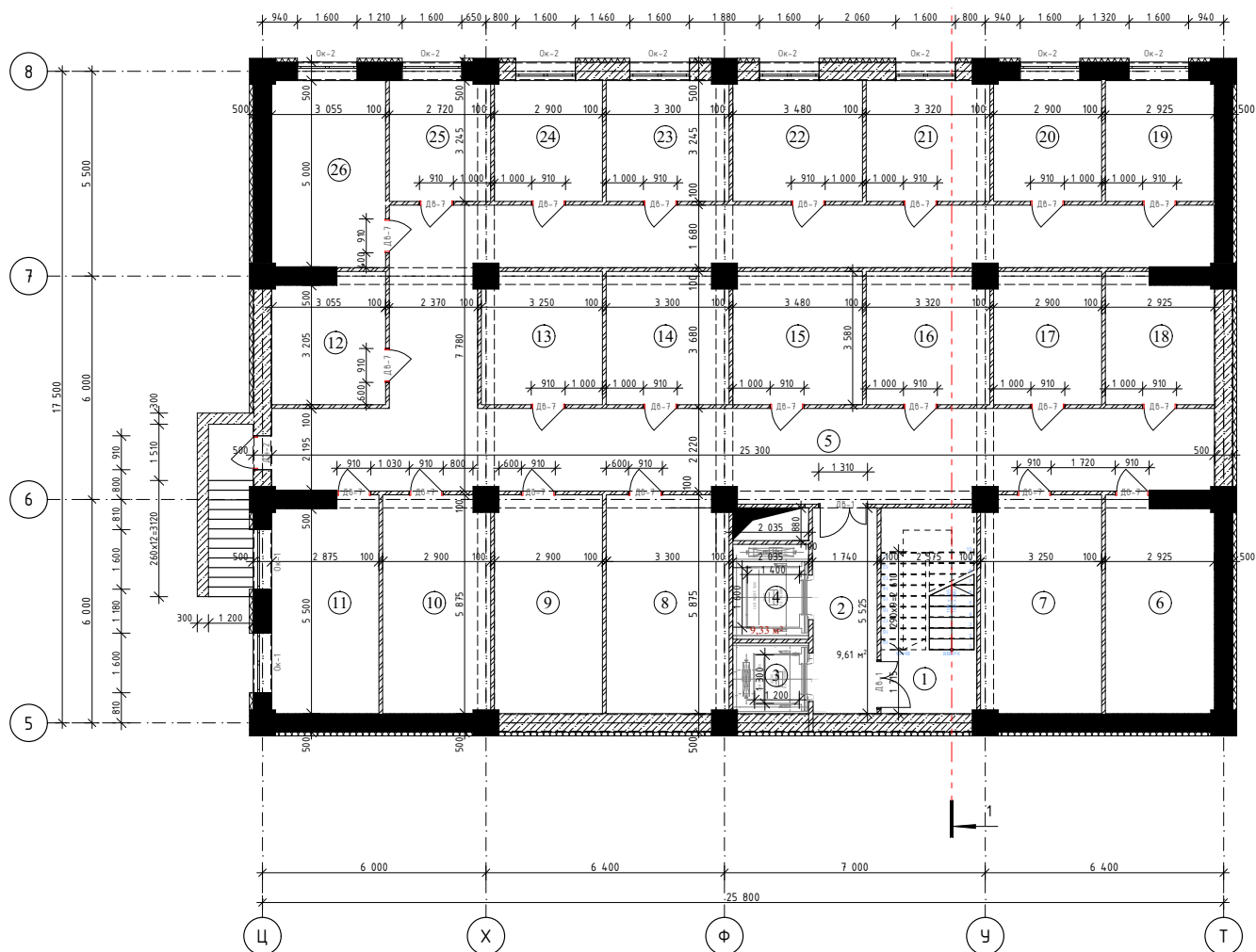
План кладового этажа (Тип-Б)
