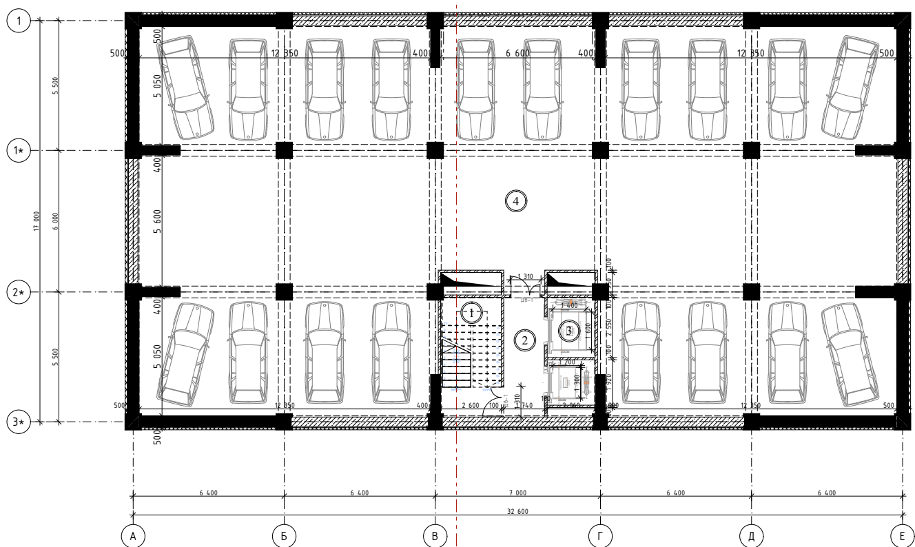
План кладового этажа (Тип-Г)
