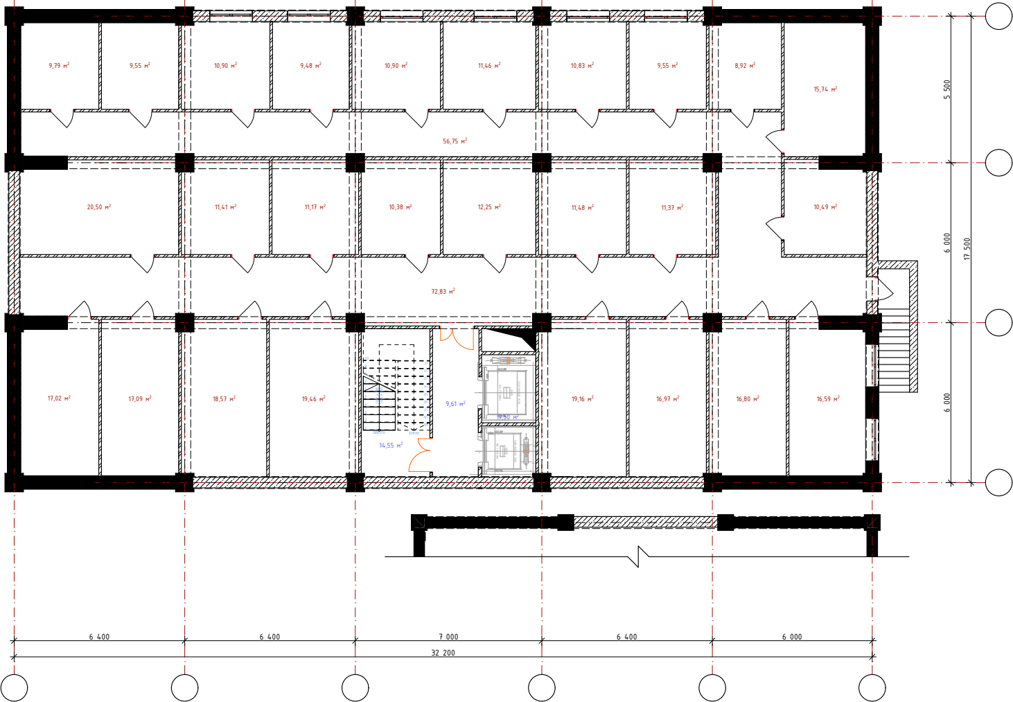
План кладового этажа (Тип-Д)
