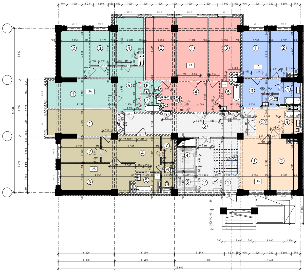
План 1-го этажа (Тип-Б)
