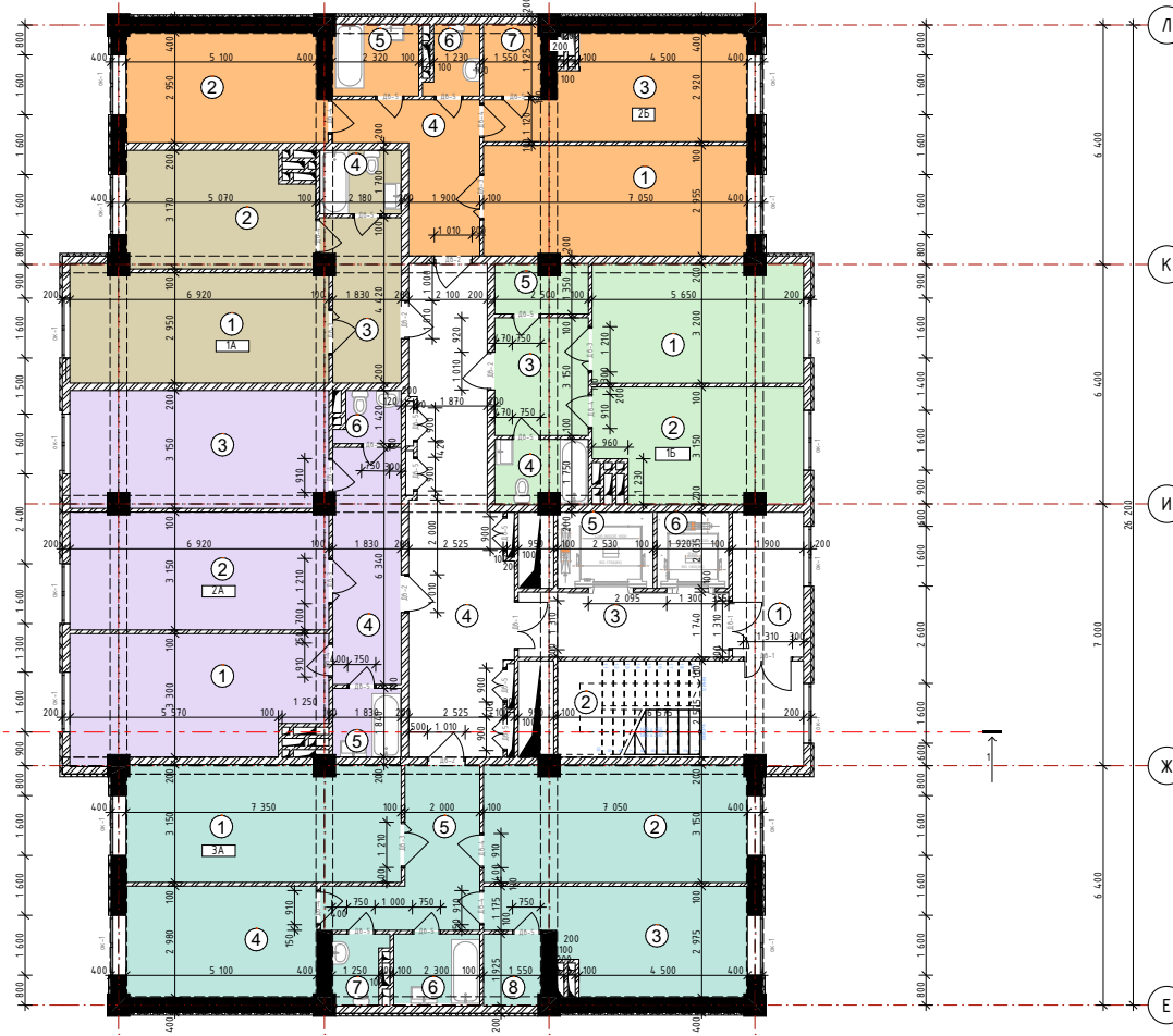
План с 2-го по 12-ый этаж (Тип-В)
