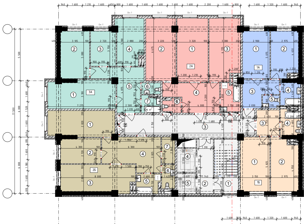
План с 2-го по 12-ый этаж (Тип-Б)
