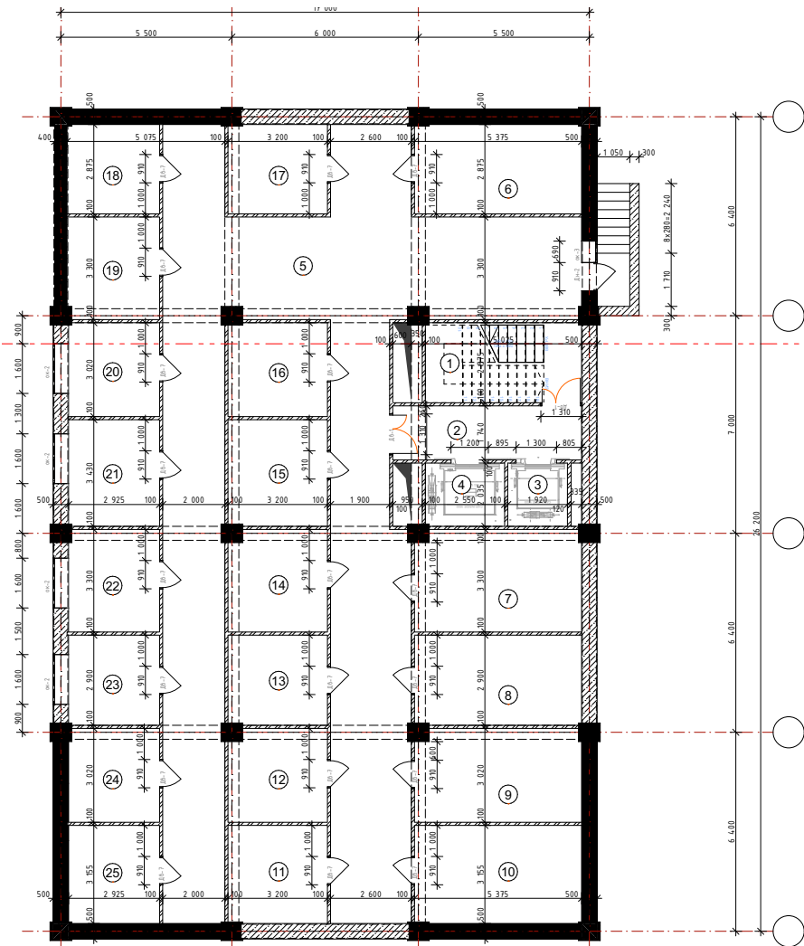
План кладового этажа (Тип-В)
