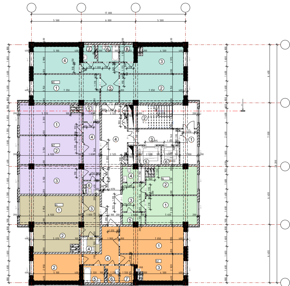
План с 2-го по 12-ый этаж (Тип-В)
