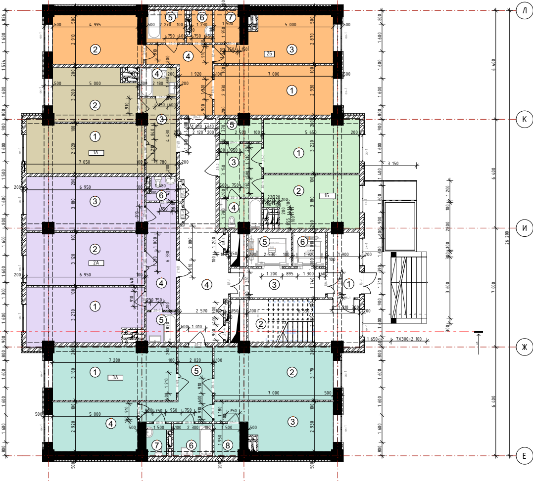
План с 2-го по 12-ый этаж (Тип-В)
