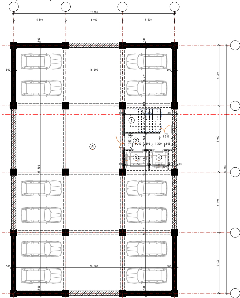
План кладового этажа (Тип-В)
