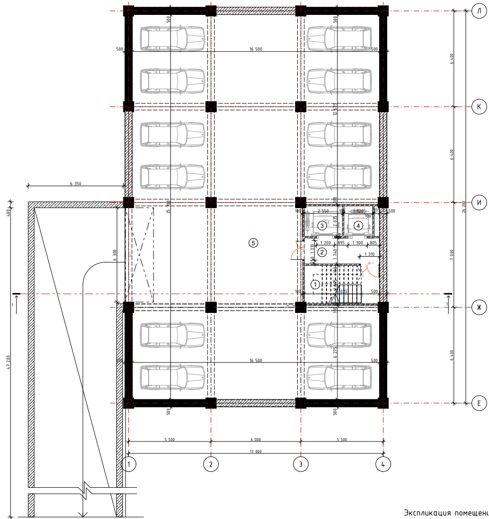
Экспликация помещений
