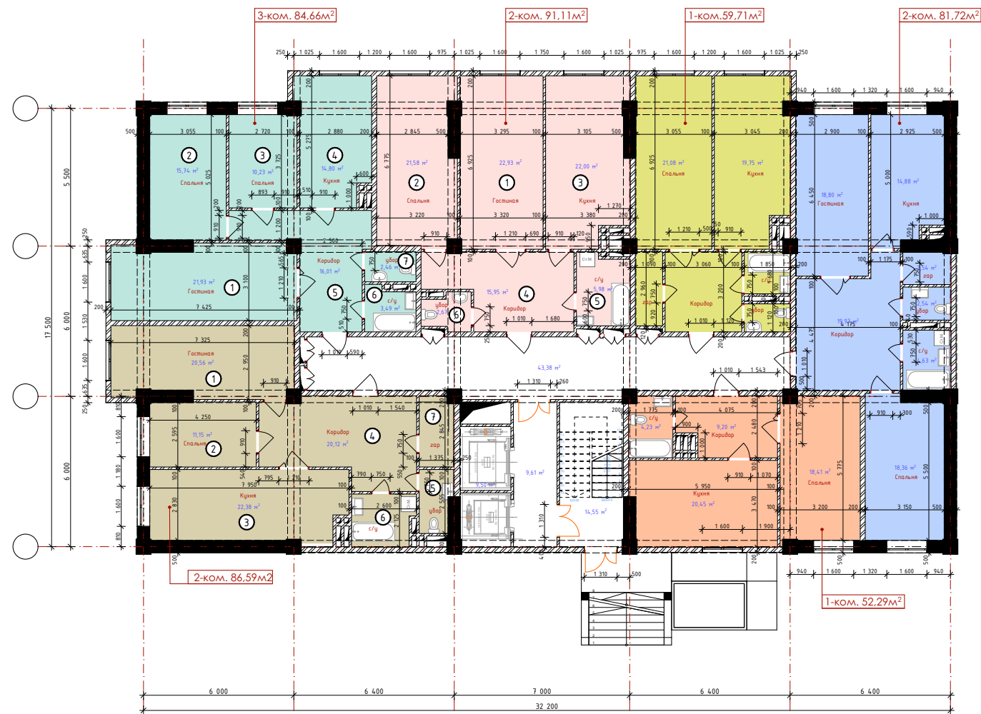
План с 2-го по 12-ый этаж (Тип-Д)
