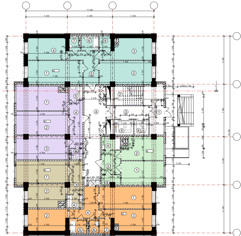
План 1-го этажа (Тип-В)
