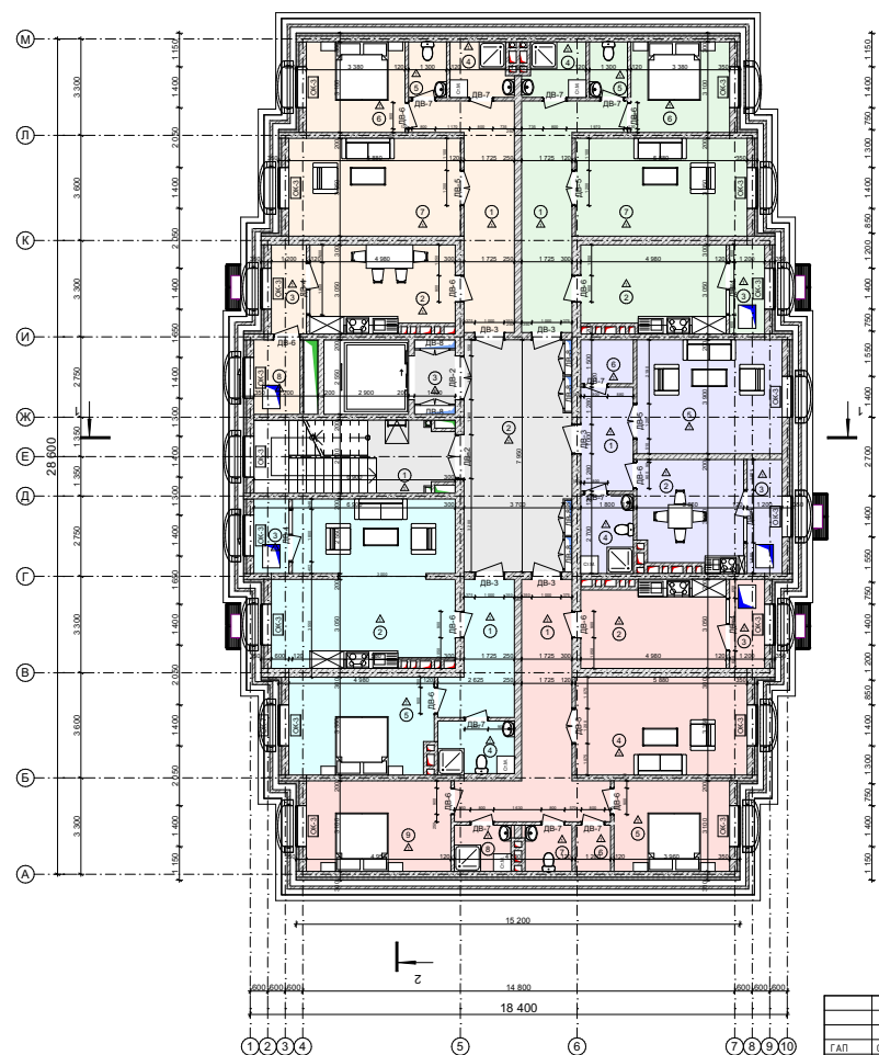
План мансардного этажа (Тип-4) 20-21-22
