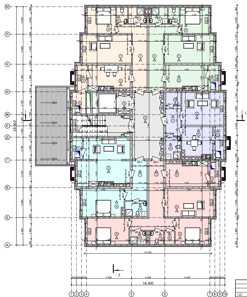
План мансардного этажа (Тип-4) 20-21-22
