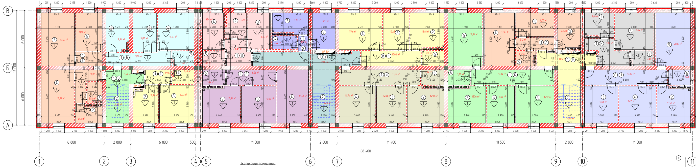
Экспликация помещений
