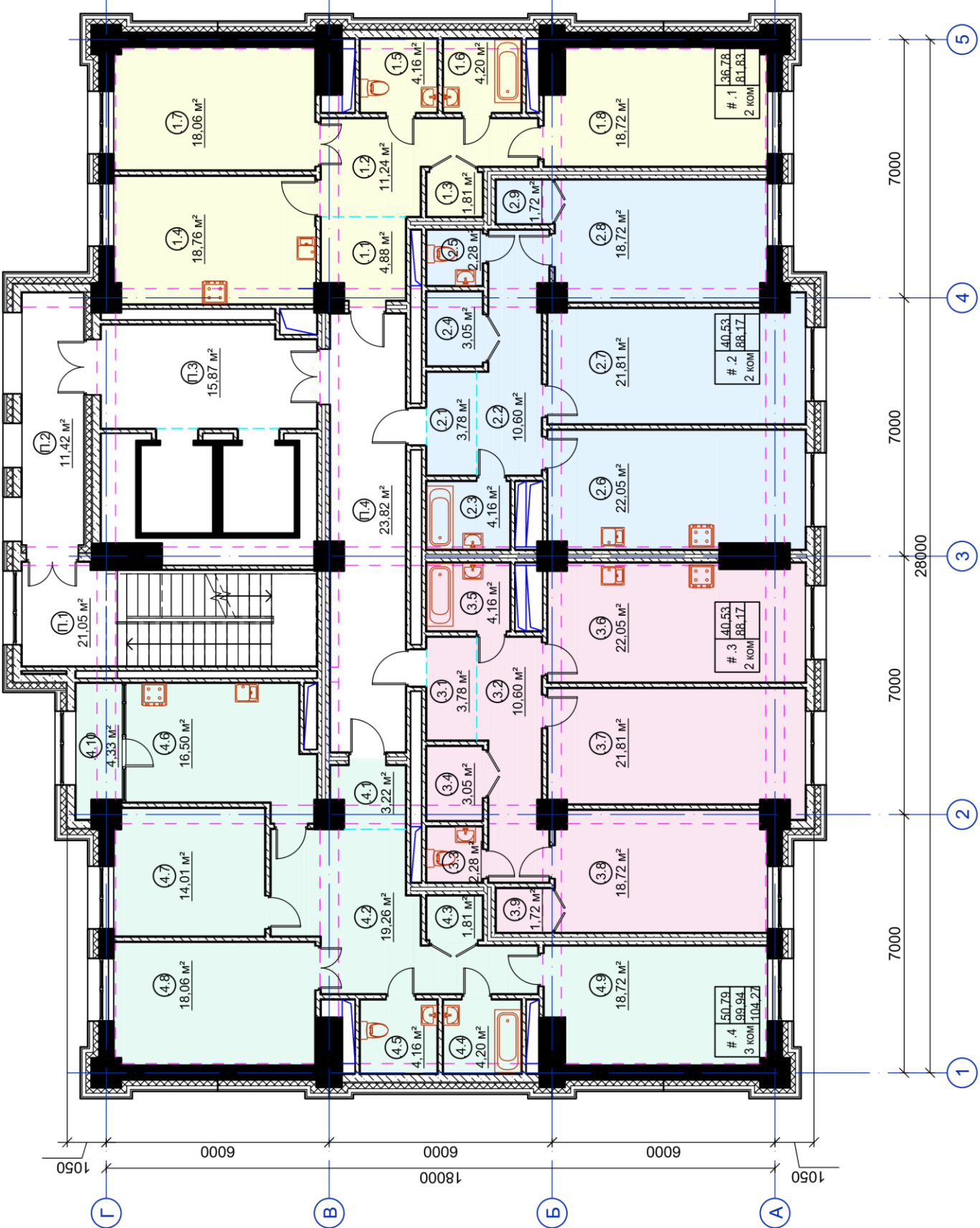
ПЛАН 3го БЛОКА план тип 1
