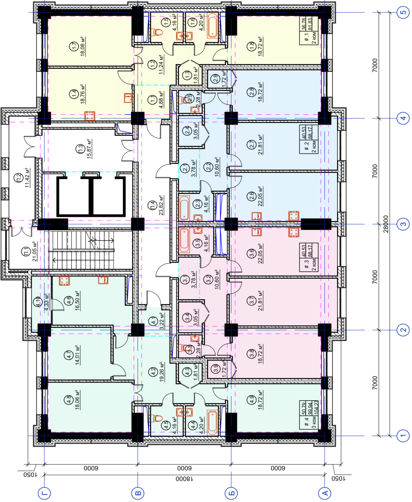
ПЛАН 6го БЛОКА план тип 1
